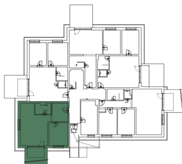
PÔDORYS
