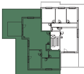
PÔDORYS
